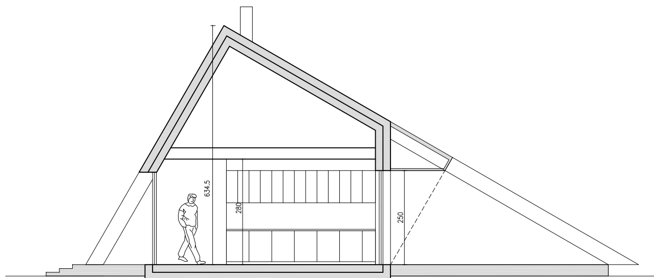
PRZEKRÓJ A-A
